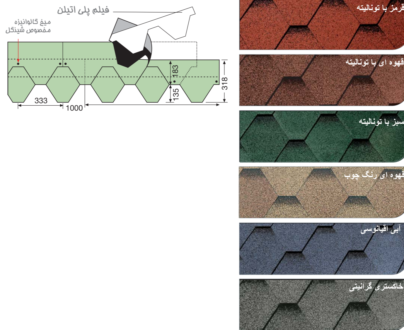
باردولین نوا (S) مطابقت مشخصات فنی و عملکرد آن در شرایط مختلف جوی طبق Class 1 استاندارد فوق توسط مؤسسات معتبر اروپائی تأیید شده است.
